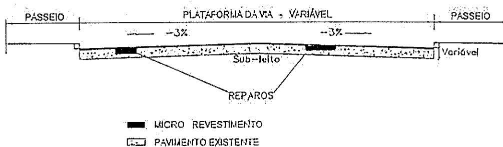
Figura 1 – Seção tipo de aplicação de micro revestimento
